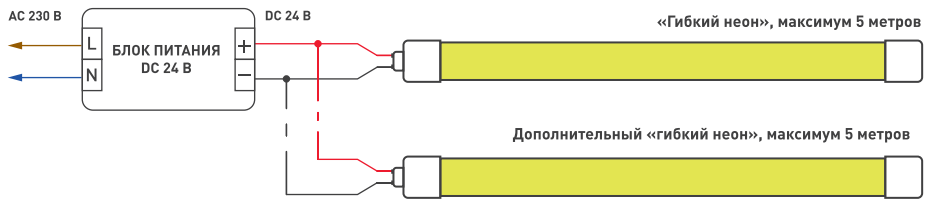
Схема 1. Подключение «гибкого неона»
