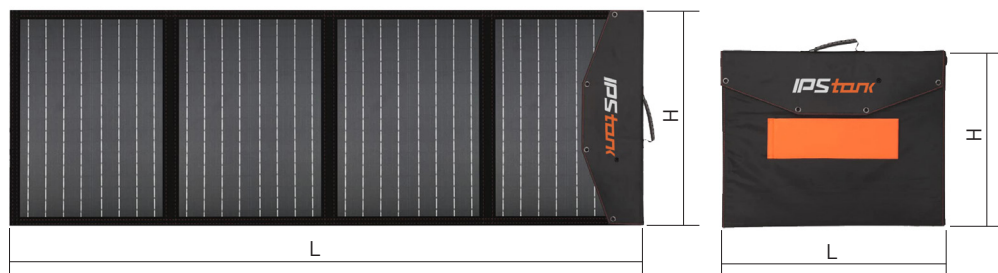
Рис. 1. Габаритные размеры
